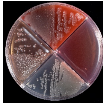
Pseudomonas spp.
