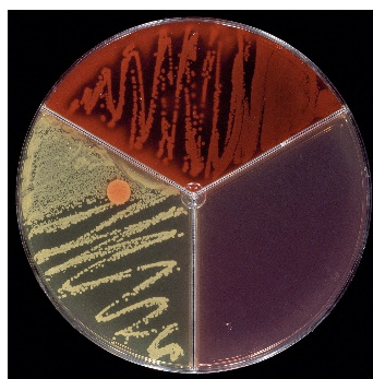
Staphylococcus aureus Pc:as + (underifrån)
