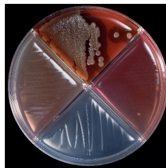
Bacillus cereus
