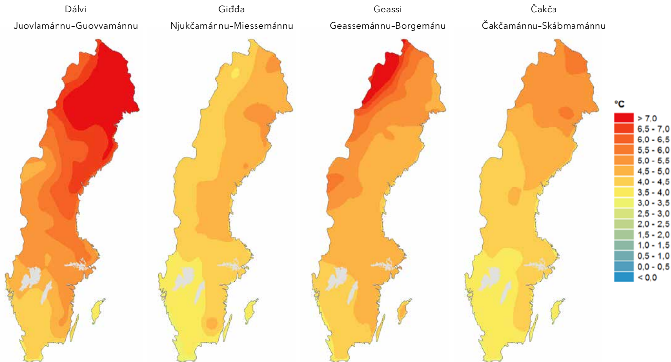
GOVVA 4. Rievdadus gaskamearálaš temperaturvrras (grádalohku) vuosáhusas RCP 8.5, čuohtilogi loahpas (2069–2098) buohtalaston referensaáigodagas (jagiin 1961–1990). Gáldu SMHI.
